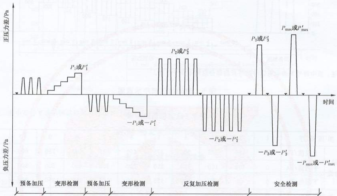
图 6 检测加压顺序示意图
