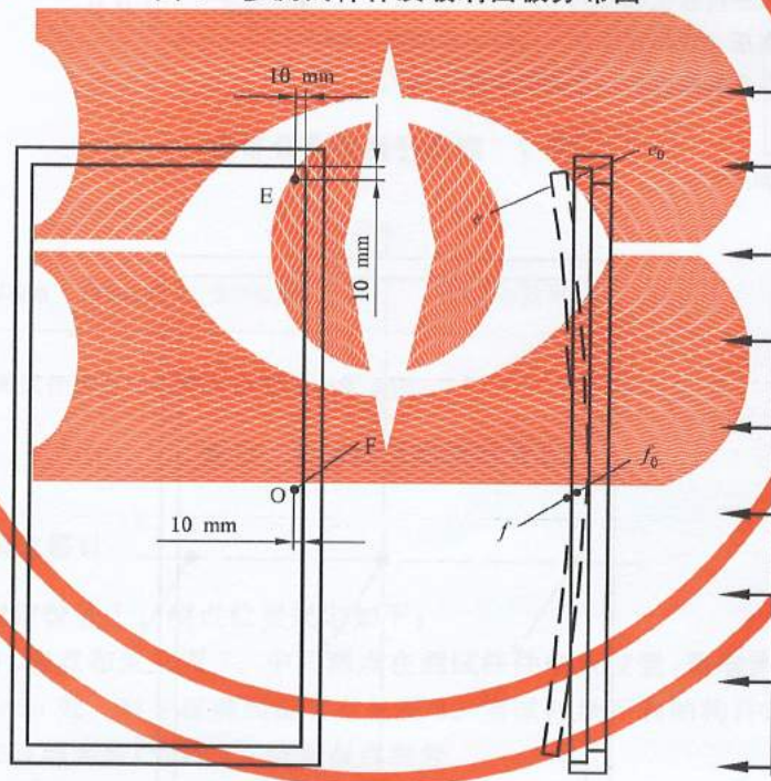
图9 多测试杆件及玻璃面板分布图
